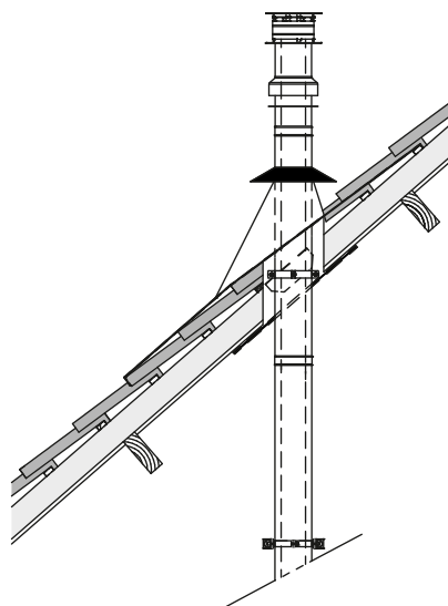
Dakdoorvoer schuin dak
