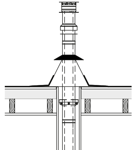
Dakdoorvoer plat dak
